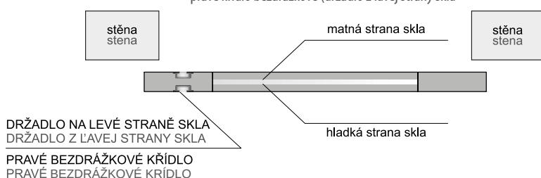
pravé bezdrážkové křídlo (držadlo na levé straně skla) pravé křídlo bezdrážkové (držadlo z ľavej strany skla)
